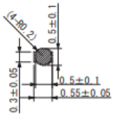
A-A'横截面(20/1)
