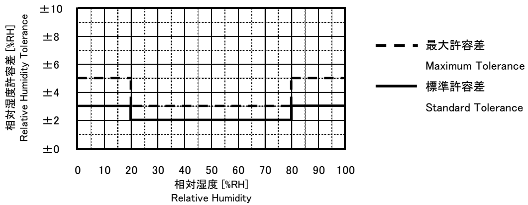
図7-1. 相对湿度測定精度許容差(25°C)
