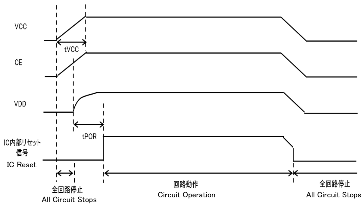
図 9-2. 起動終了シーケンス(電源制御)
