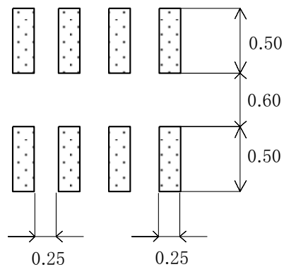
ランド詳細図 (A、B 基板共通)
