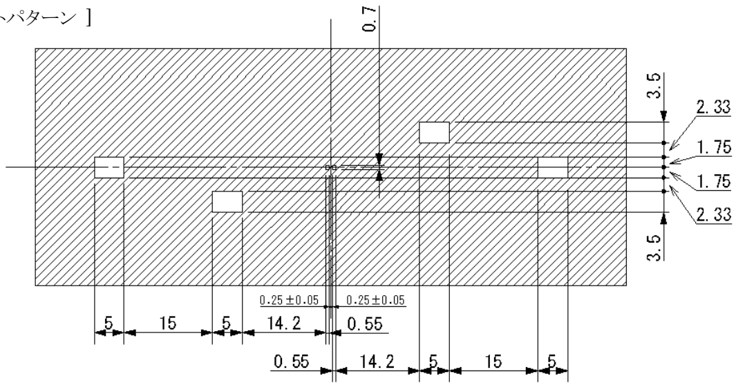
[銅箔パターン]
