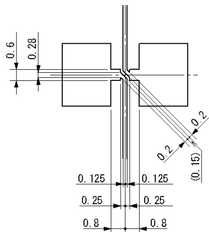
[銅箔ランドパターン]
