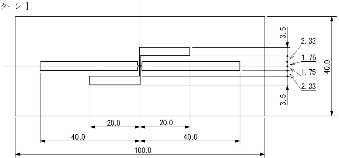
[銅箔ランドパターン]
