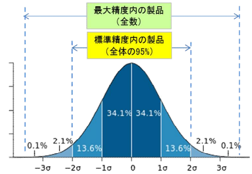
図4-1. 精度分布
