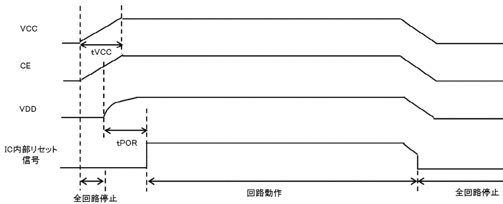
図 9-2. 起動/終了シーケンス(電源制御)
