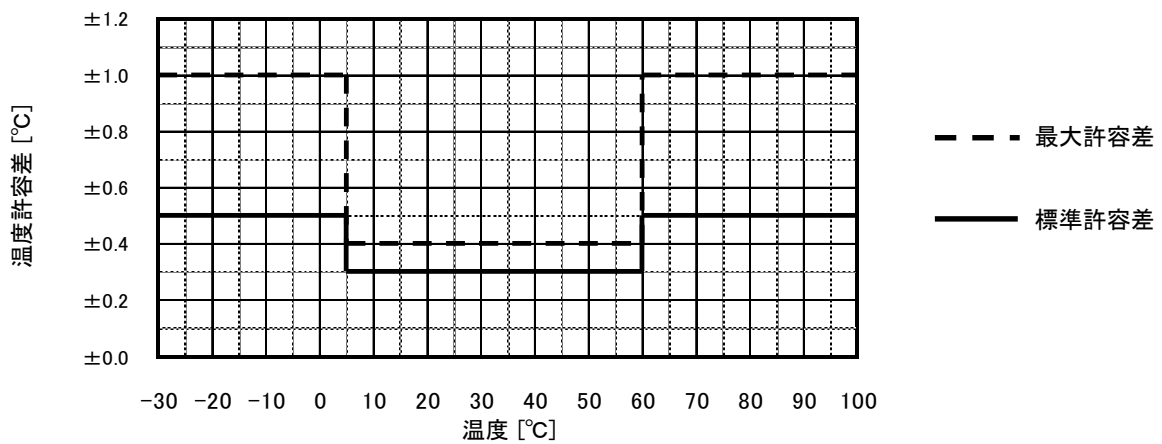
図7-3. 温度測定許容差
