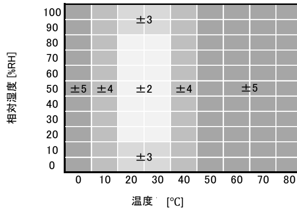
図7-2. 温度範囲(0~80°C)における相对湿度の測定精度
