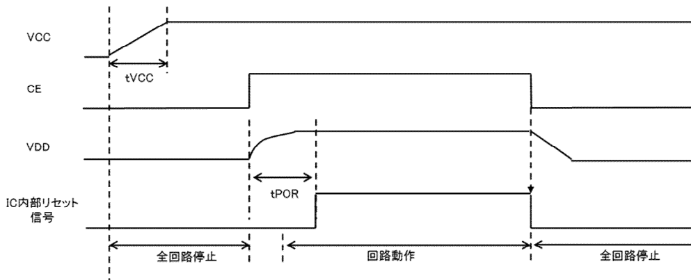
図 9-1. 起動/終了シーケンス(CE制御)
