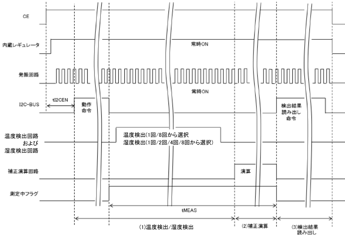
図 9-3. 温度/湿度検出シーケンス
