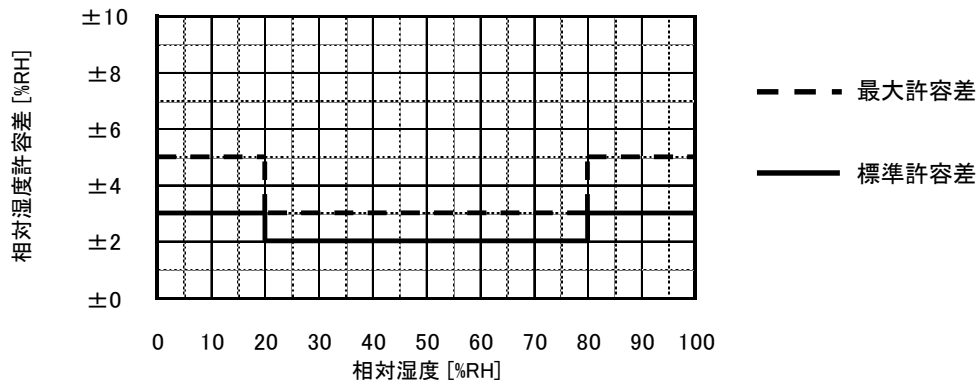
図7-1. 相对湿度測定精度許容差(25°C)
