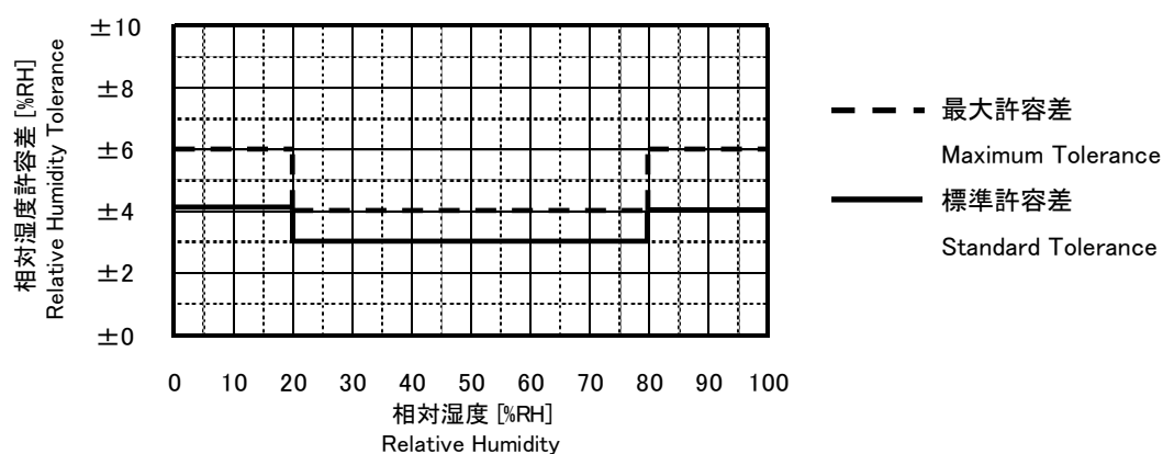
図6-1. 相对湿度測定精度許容差(25°C)
