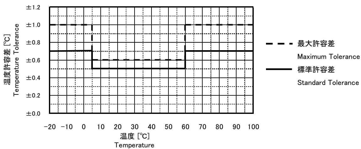
図6-3. 温度測定許容差
