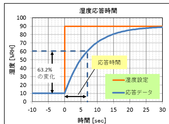
図4-3. 応答時間の定義
