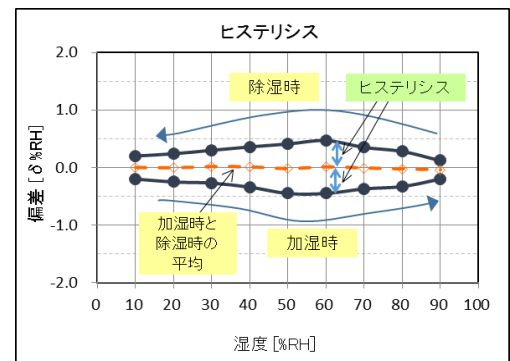
図4-4. ヒステリシスの定義
