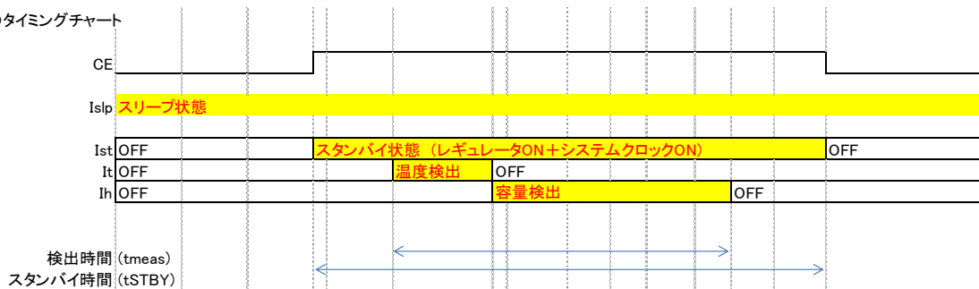
図4-2. 測定タイミングチャート
