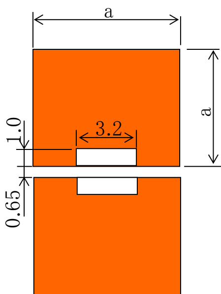
銅箔寸法
